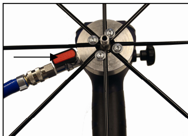
Abb. 65: Robinet ouvert
