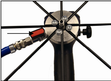
Abb. 14: Absperrhahn Druckluft geöffnet
